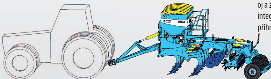
Digger P FW | doplňkový nosič s nápravou, zásobník hnojiva, přihnojování do 2 horizontů
